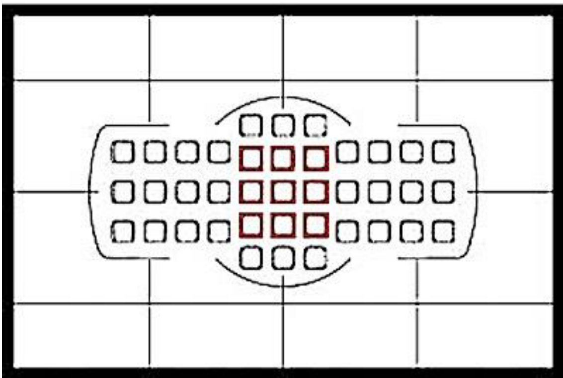
Module AF à 39 collimateurs/points Nikon
